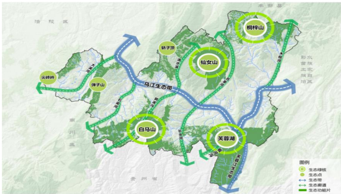
图3 生态格局图
