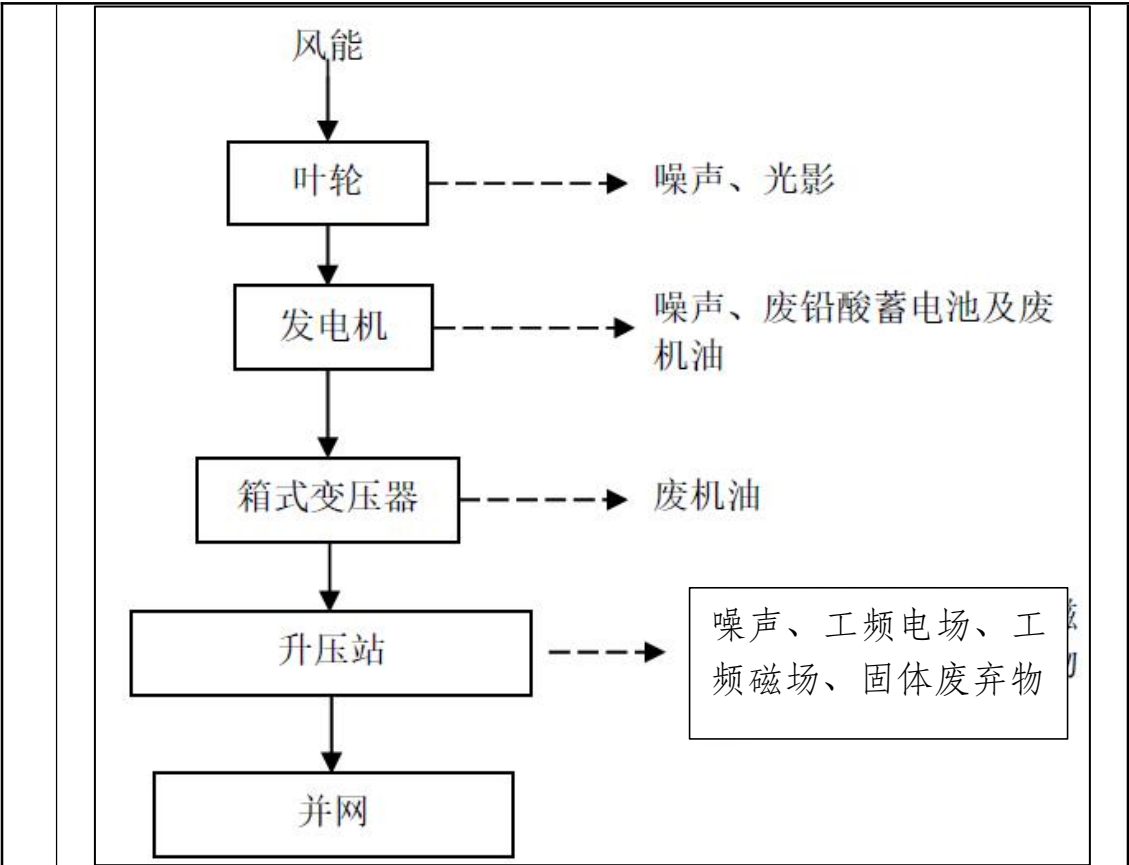
图 4-2 本工程运营期发电工艺流程与产污环节图
