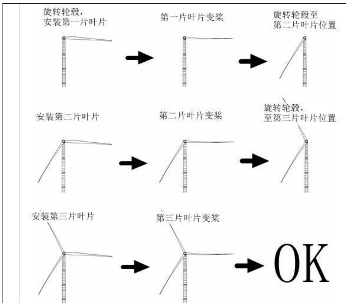
图 2-1 单叶片吊装流程图
