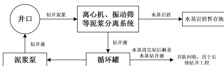
图 5-1 本项目钻井过程中钻井液循环方式图
